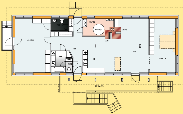
Esimerkkitalon pohjapiirros ja varaajan ja tulisijan sijoitus rakennuksessa. Lähde: Pekka Leppänen
