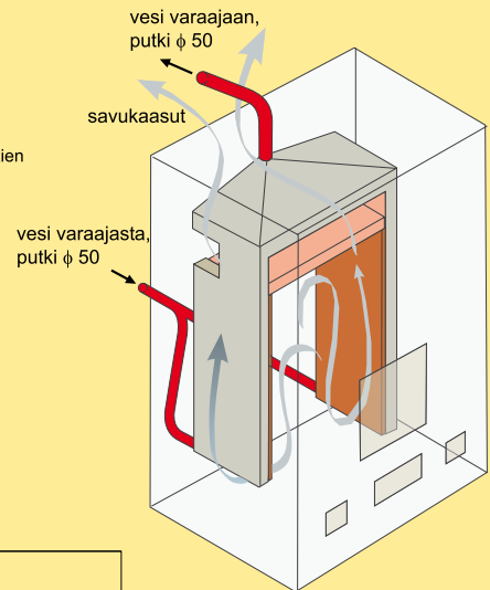
Lämmönvaihtimen sijoittaminen tulisijaan. Lähde: Pekka Leppänen
